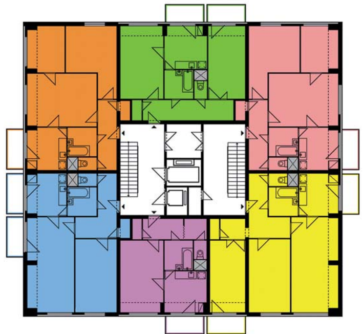
PŮDORYS typického podlaží – povšimněte si dvou schodišť.
