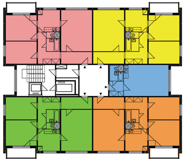
DISPOZICE typického podlaží.
