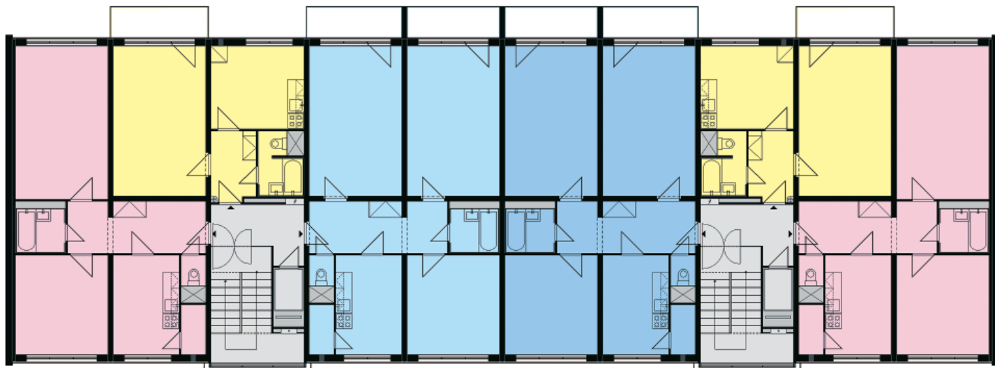
PŮDORYS typického podlaží dvojdomu T06B-OS 70.
