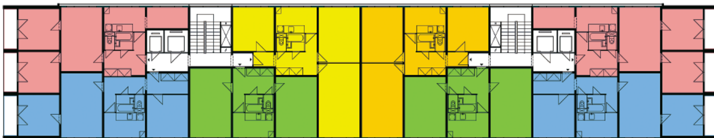
TYPICKÉ PODLAŽÍ panelového domu G-OS.
