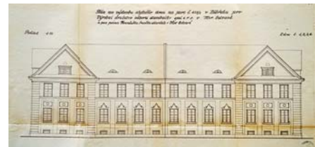
Návrh uličního průčelí domů na Krokové ulici v Zábřehu nad Odrou, A. Korner, 1926
