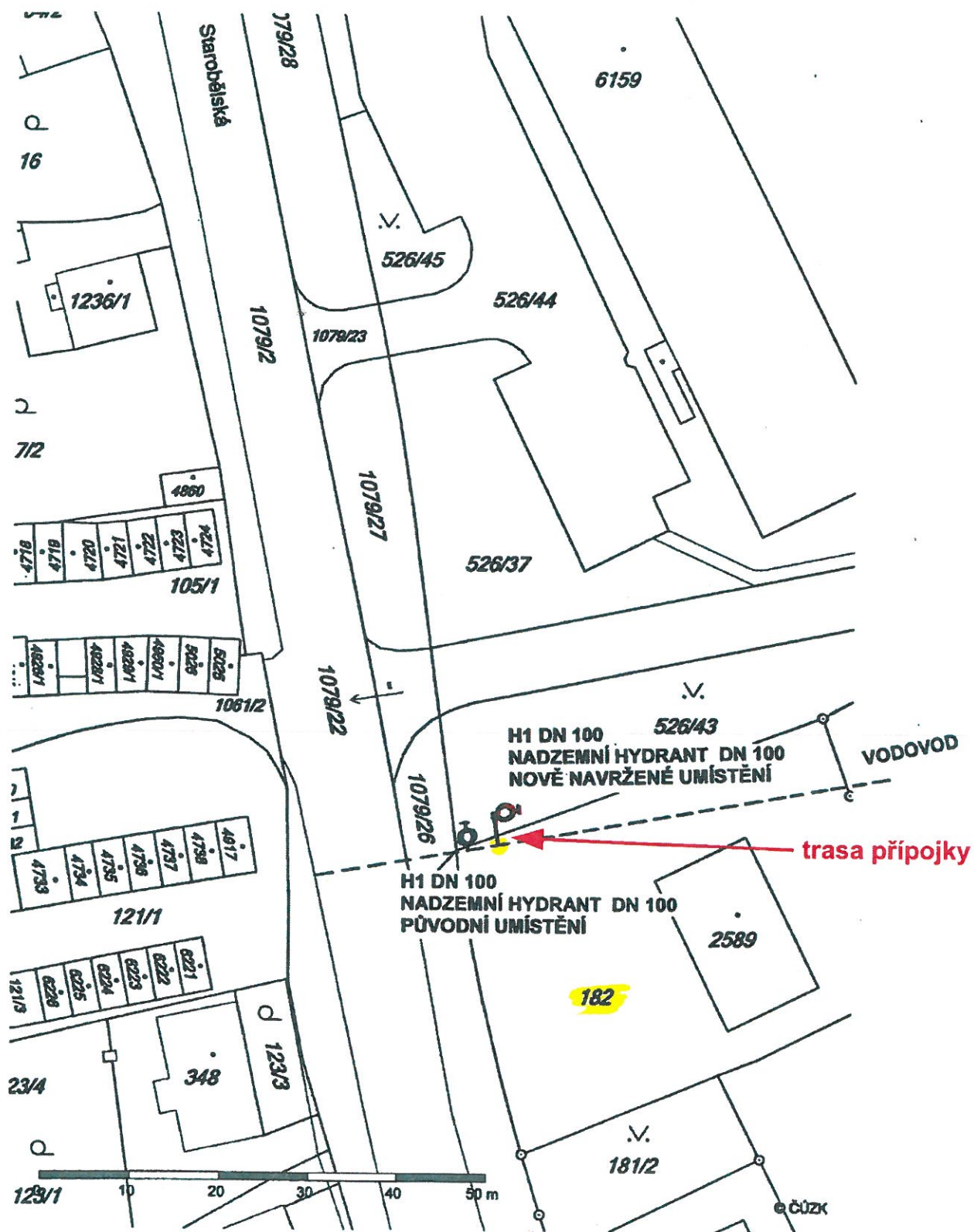
ATLETICKÁ HALA VÍTKOVICE SO 02.9 ÚPRAVA A PŘELOŽKA NADZEMNÍHO HYDRANTU SITUACE
